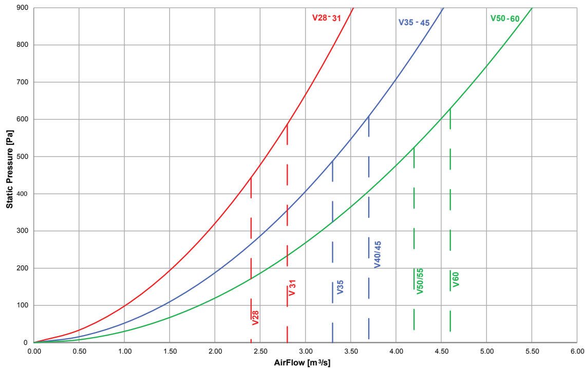
V28-60 - EC Forward Fan Curve
